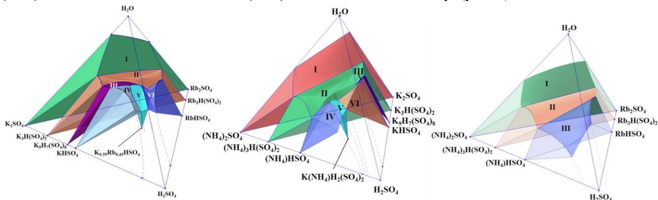
Рисунок.1. Изометрическая проекция фазовых диаграмм K_2SO_4-Rb_2SO_4-H_2SO_4-H_2O , K_2SO_4-(NH_4)_2SO_4-H_2SO_4-H_2O и Rb_2SO_4-(NH_4)_2SO_4-H_2SO_4-H_2O .
