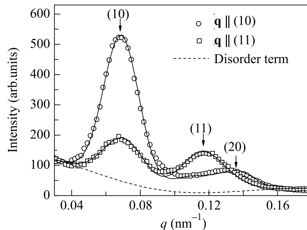
Рис.3. Зависимость интенсивности нейтронного рассеяния от переданного импульса I(q) для образца, обладающего высокоупорядоченной структурой пор (ААО3), при \mathbf{q} \parallel (10) и \mathbf{q} \parallel (11)
