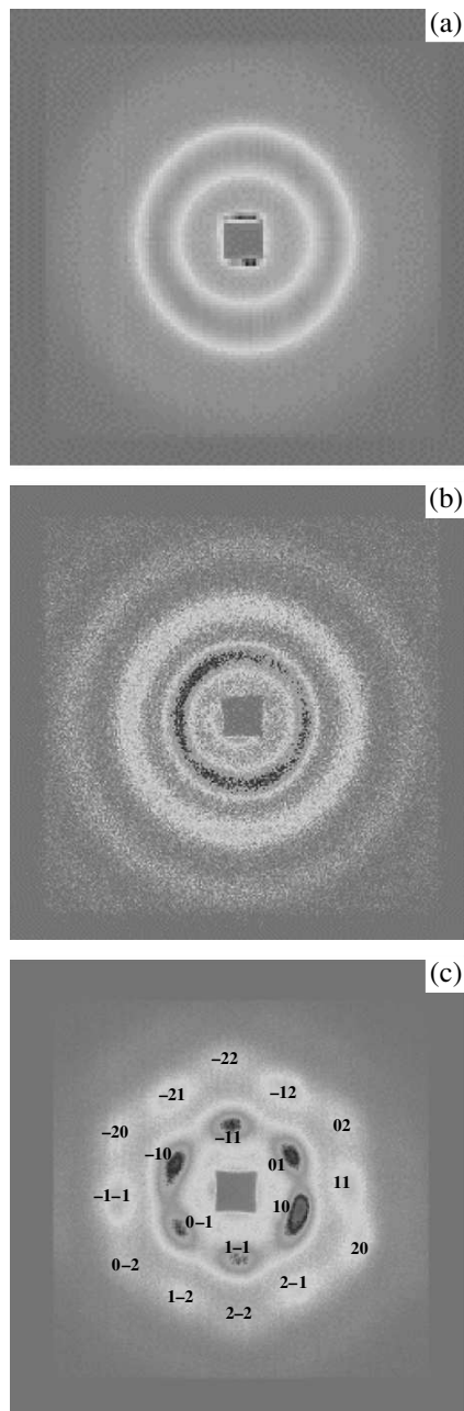
Рис.2. Карты интенсивности малоуглового рассеяния нейтронов для: (а) образца, изготовленного из технического алюминия (ААО1), (б) образца из высокочистого алюминия с мелкозернистой микроструктурой (ААО2), и (с) образца из высокочистого алюминия с крупнозернистой микроструктурой (ААО3)
